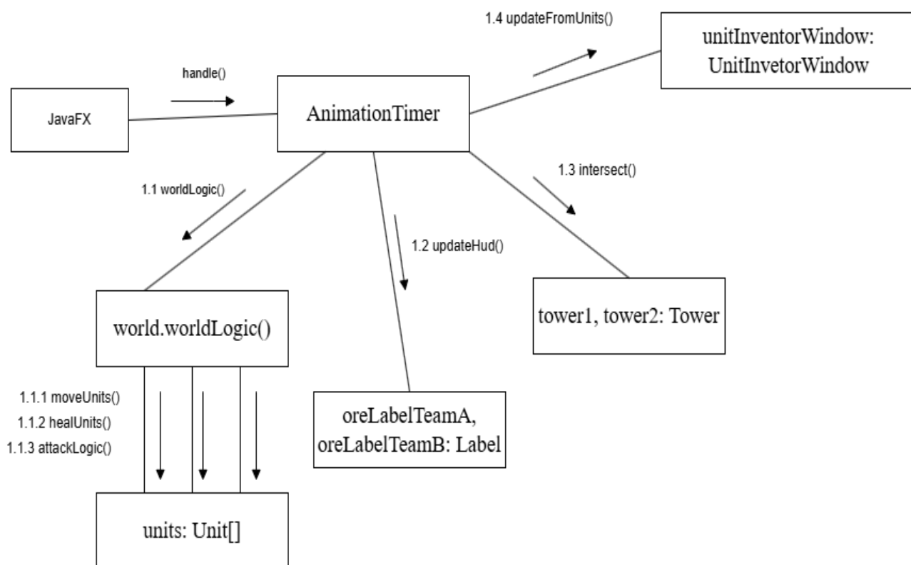
Рисунок 3.5 – Діаграма кооперації
