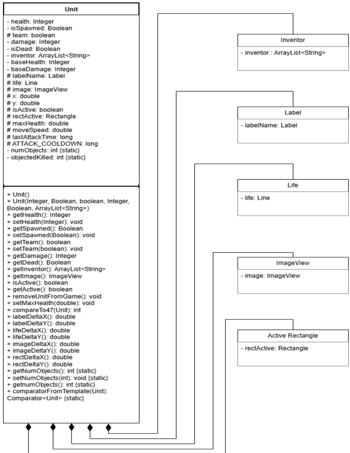
Рисунок 3.3 – Діаграма композиції
