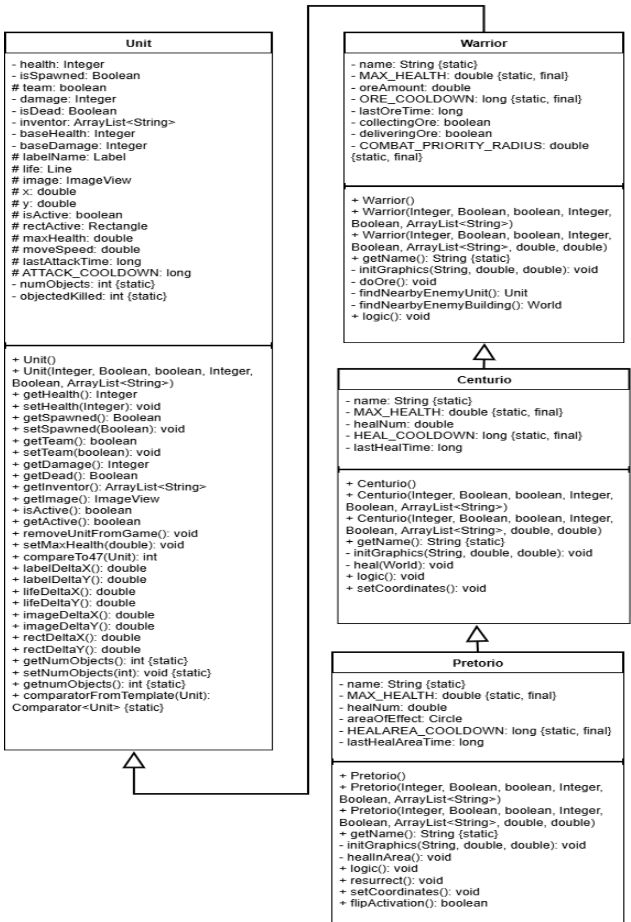
Рисунок 3.1 – Діаграма наслідування
