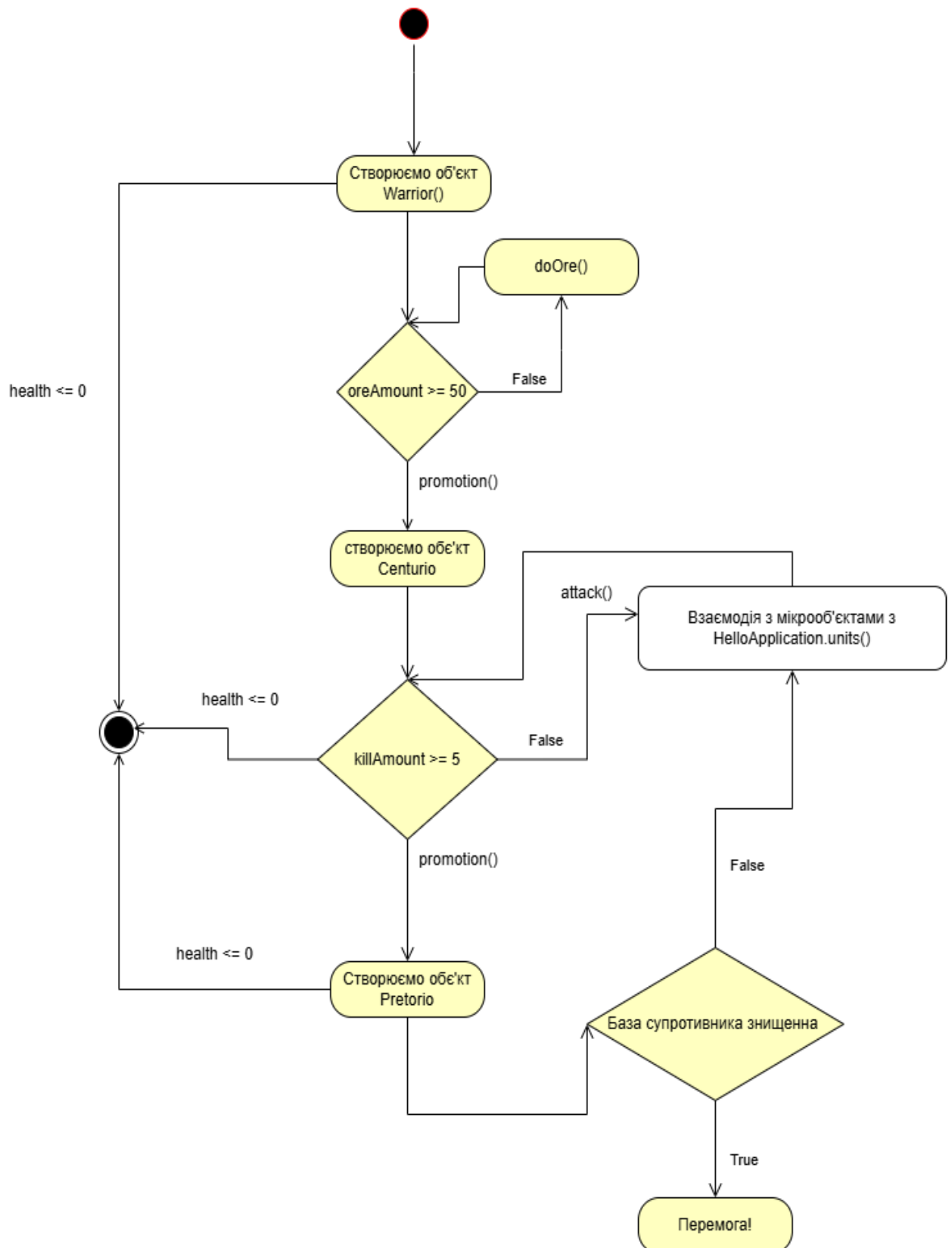
Рисунок 3.7 – Діаграма станів
