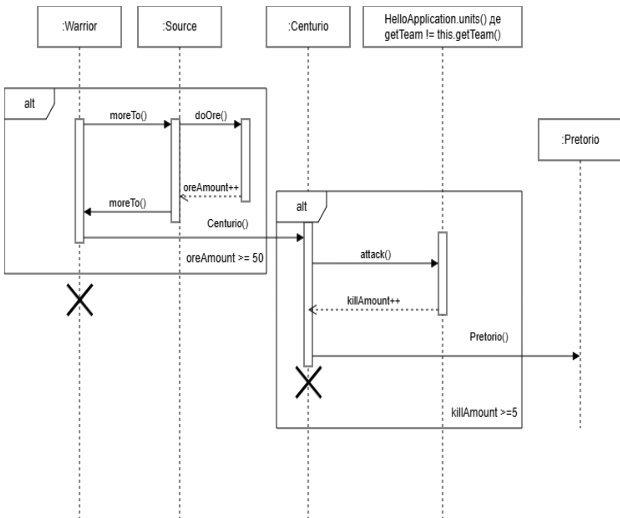
Рисунок 3.6 – Діаграма послідовності
